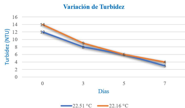
Fig. 5 Relación de los días de tratamiento y la reducción de la turbidez
