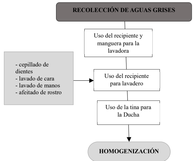
Fig 3. Esquema de recolección de aguas grises
