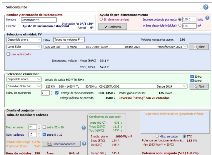
FIGURA 5: Modelado del sistema fotovoltaico en PVsyst.
