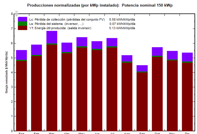
FIGURA 8: Producción normalizada de kWp instalada.
