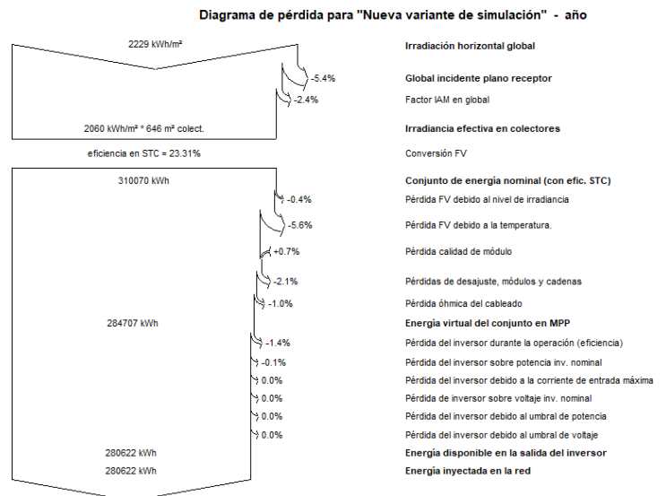
FIGURA 10: Diagrama de pérdidas a lo largo de todo el año.
