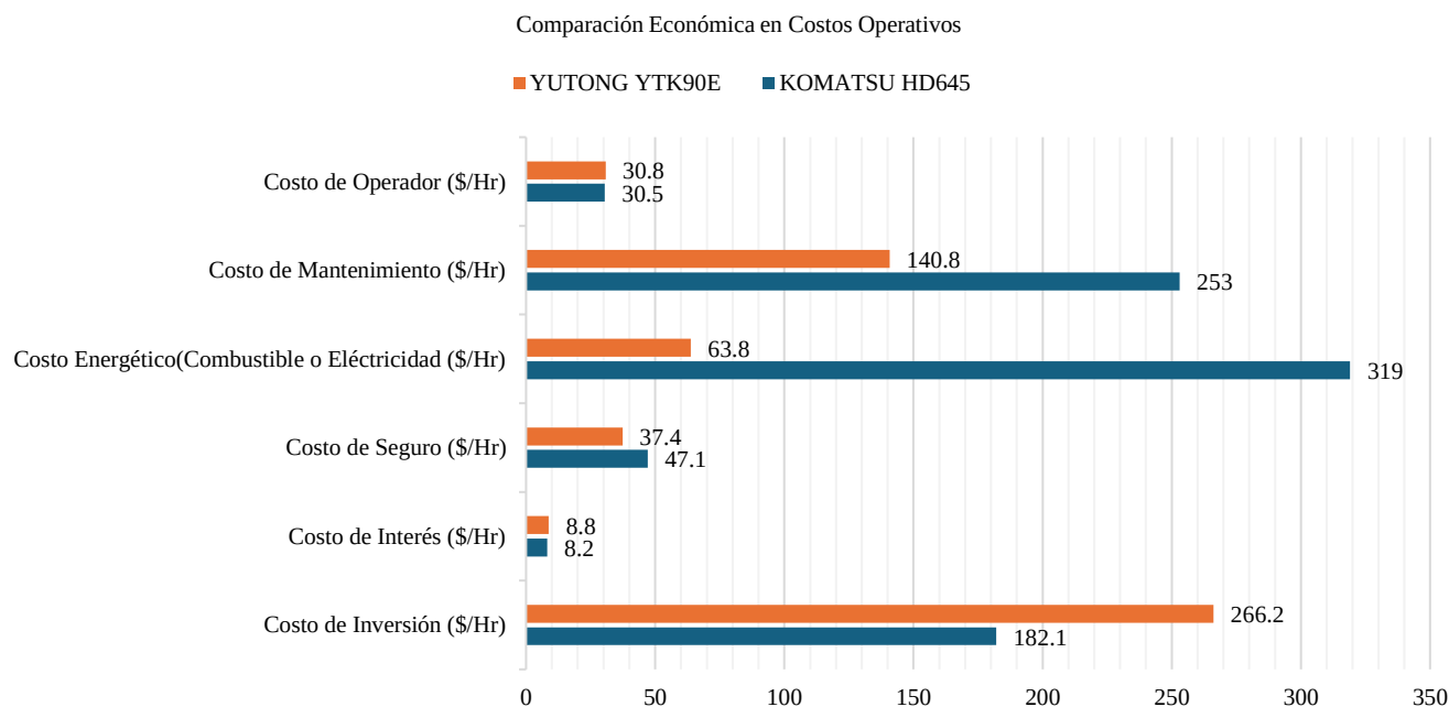
Fig. 8. Comparación económica según los costos operativos de camiones diésel y eléctricos. Fuente: Propia.
