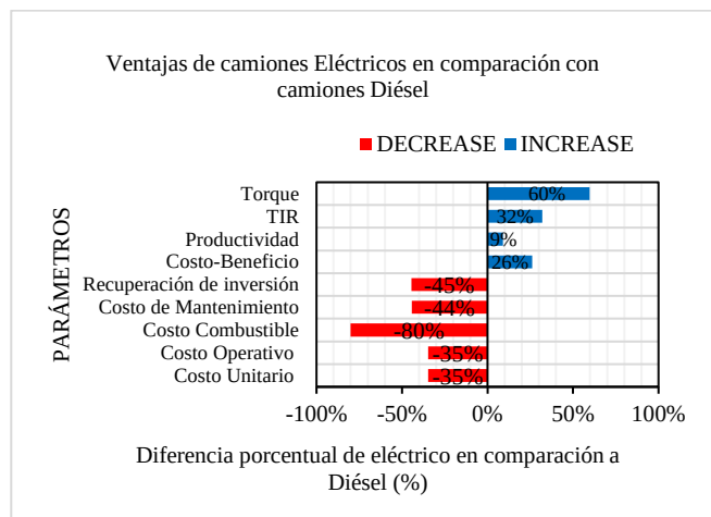
Fig. 13. Ventajas comparativas de camiones Diesel y eléctricos. Fuente: Propia.
