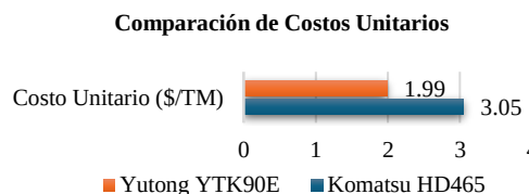
Fig. 9. Comparación de costos unitarios de acarreo. Fuente: Propia.
