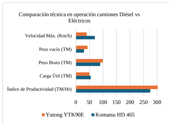
Fig. 7. Comparación técnica en operación de camiones diésel y eléctricos. Fuente: Propia.
