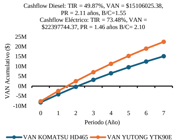
Fig. 12. Comparación económica financiera de ambos proyectos de inversión. Fuente: Propia.
