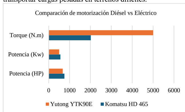
Fig. 6. Comparación de características de motorización de camiones diésel y eléctricos. Fuente: Propia.
