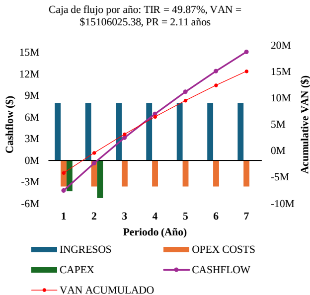
Fig. 10. Flujo financiero de camiones Diésel Fuente: Propia
