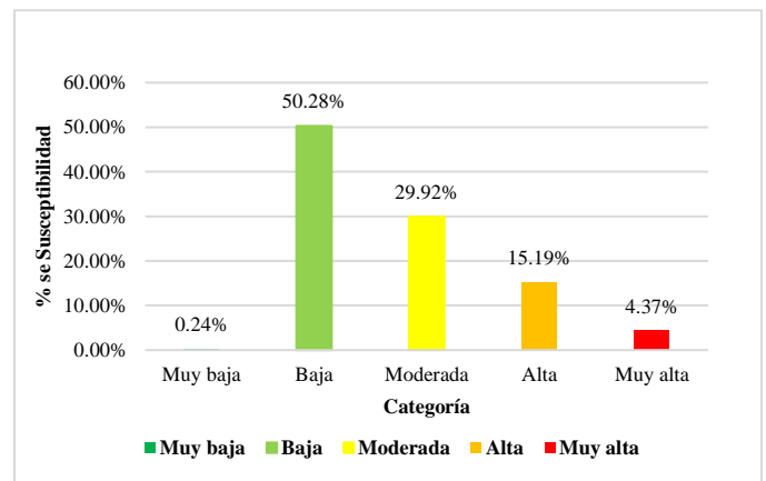
Fig. 9 Categorías de susceptibilidad a erosión hídrica.
