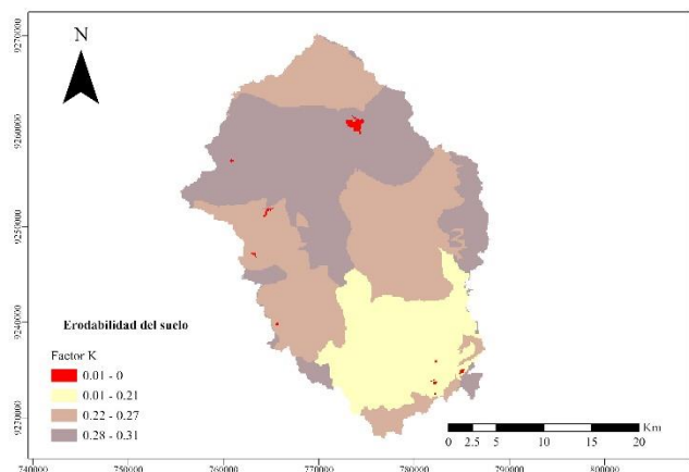
Fig. 3 Mapa del factor K (Erodabilidad del Suelo).
