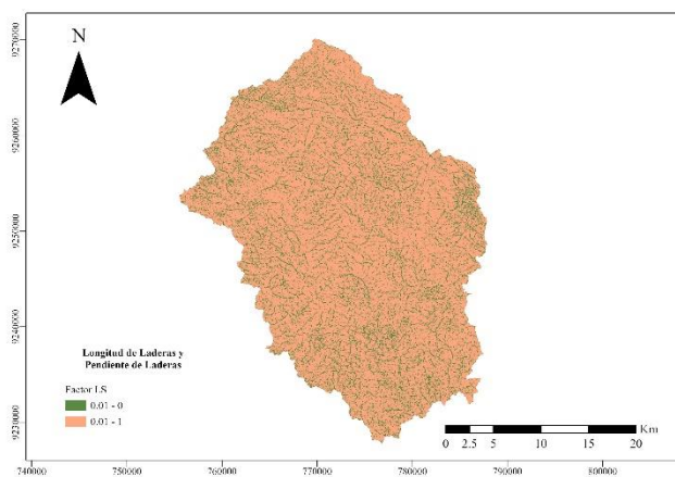
Fig. 4 Mapa del factor LS (Longitud de Ladera y Pendiente de Ladera).
