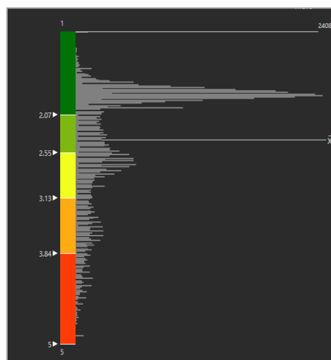
Fig. 7 Histograma de raster final con la aplicación del modelo USLE.
