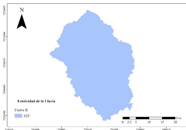
Fig. 2 Mapa del factor R (Erosividad de la Lluvia).
