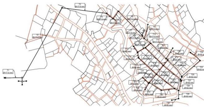
Fig. 5. Distribución de las tuberías propuestas en el software EPANET
