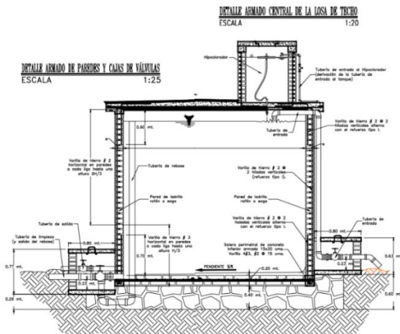
Fig. 7. Tanque propuesto.
