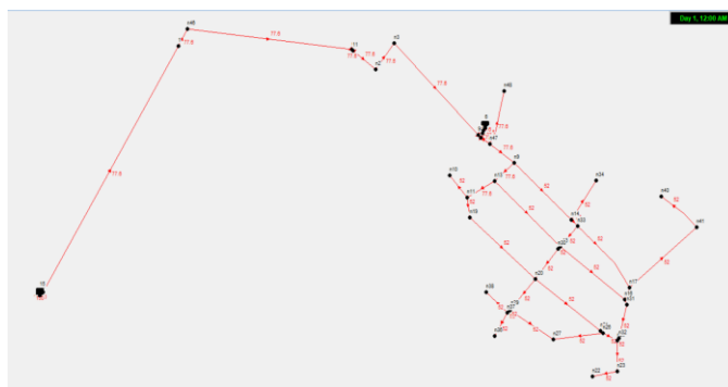
Fig. 4. Simulación de diámetro de tuberías en pulgadas según el software EPANET.
