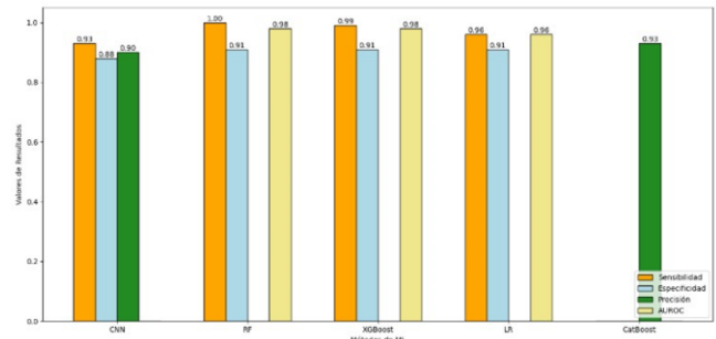
Fig 4 Mediciones de resultados por métodos de ML en personas y dispositivos portátiles
