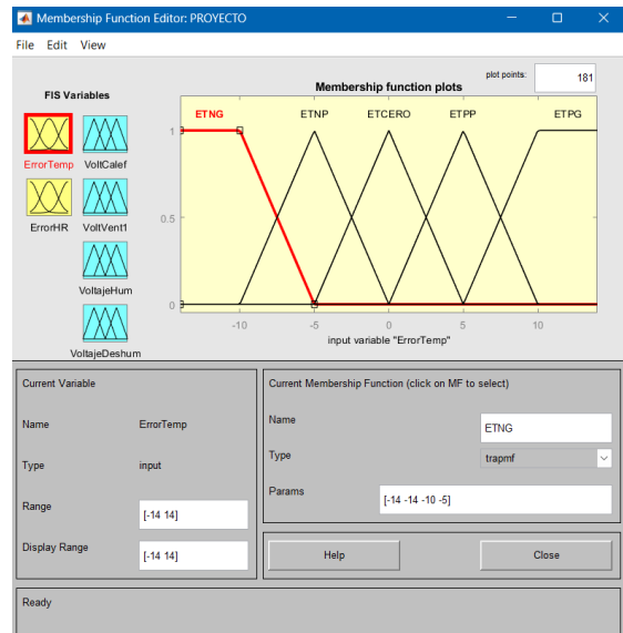
Figura 3. Conjunto difuso del error de la Temperatura en Matlab
