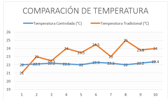
Figura 6. Comparación de temperatura controlada vs. tradicional
