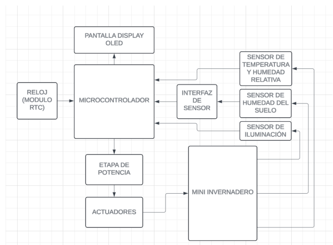
Figura 2. Diagrama de bloques de conexiones. Nota: Diagrama de bloques del monitoreo y control automático del miniinvernadero. Autoría: Propia.
