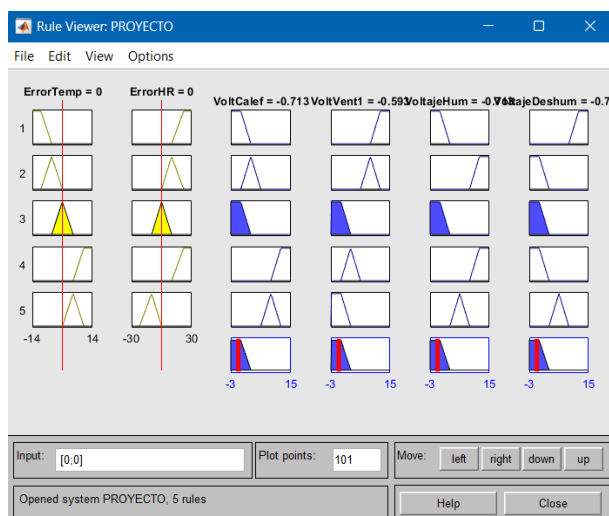
Figura 4. Visualizador de las reglas de la lógica difusa
