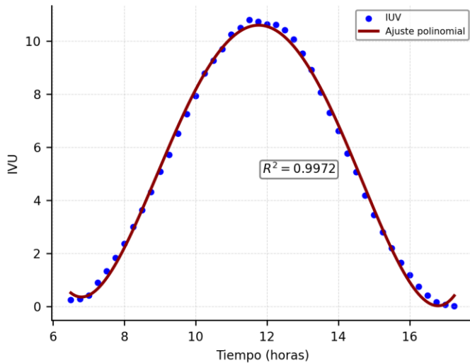
Fig. 2 Comportamiento y ajuste polinomial del IUV durante el periodo de estudio.
