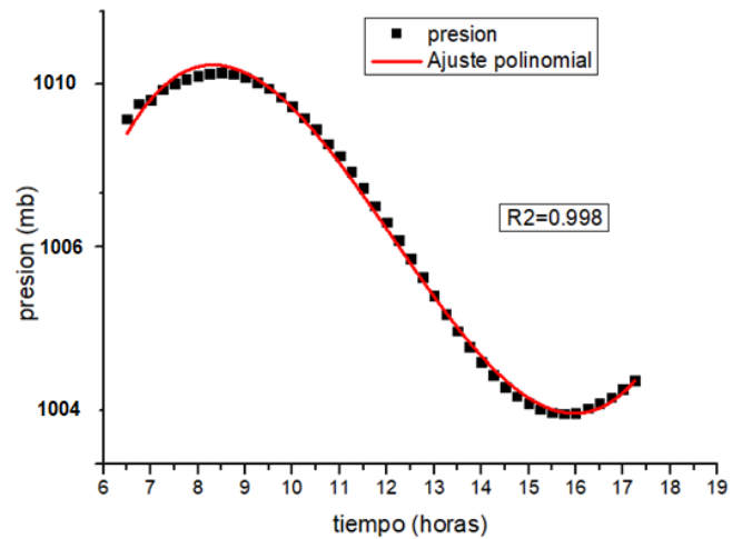
Fig. 5 Distribución diaria (entre las 6 y 18 horas) de los datos de la presión atmosférica en la ciudad de Puno durante el periodo de medición.
