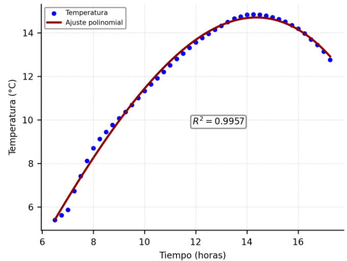
Fig. 3 Comportamiento y ajuste polinomial de la temperatura diurna durante el periodo de estudio.
