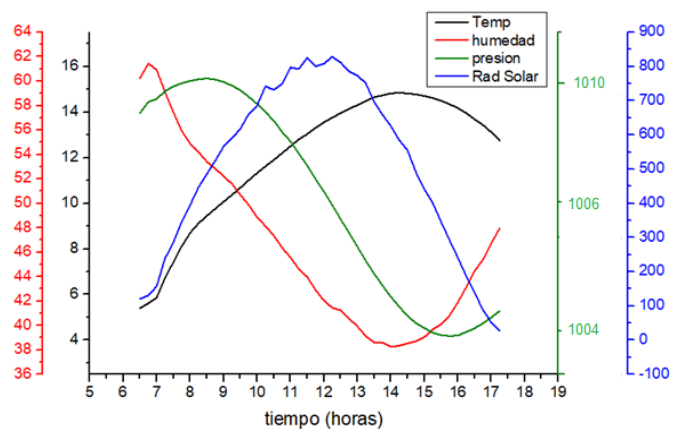
Fig. 6 Comportamiento de las variables meteorológicas entre las 6 y 18 horas durante el periodo de medición.
