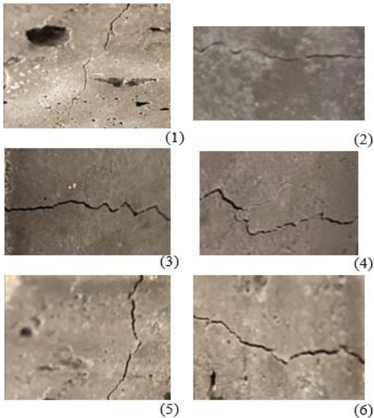
Fig. 12. Fotografías de grietas en probetas con incorporación de Bacillus subtilis que oscila entre 0.45mm a 1.41mm. (Elaboración propia)
