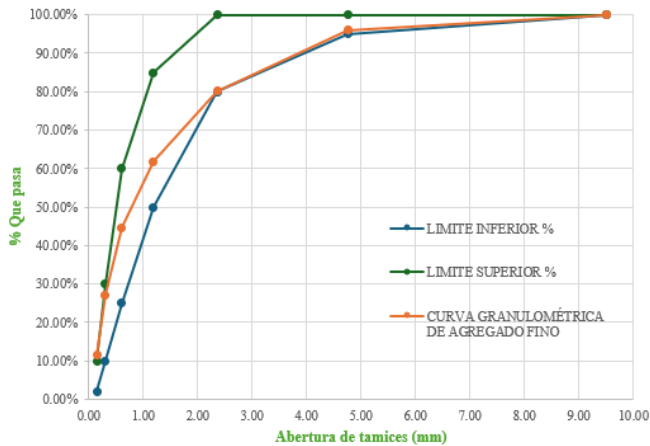
Fig. 5. Análisis granulométrico de agregado fino. (Elaboración propia)
