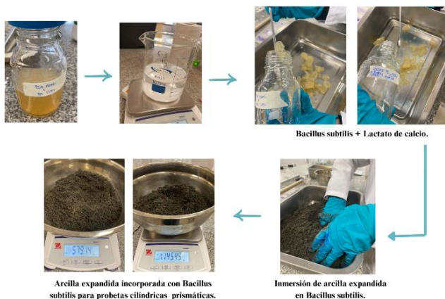
Fig. 11. Esquema de incorporación de Bacillus subtilis a la arcilla expandida. (Elaboración propia)
