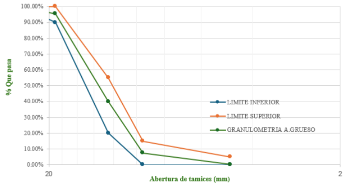
Fig. 6. Análisis granulométrico de agregado grueso. (Elaboración propia)
