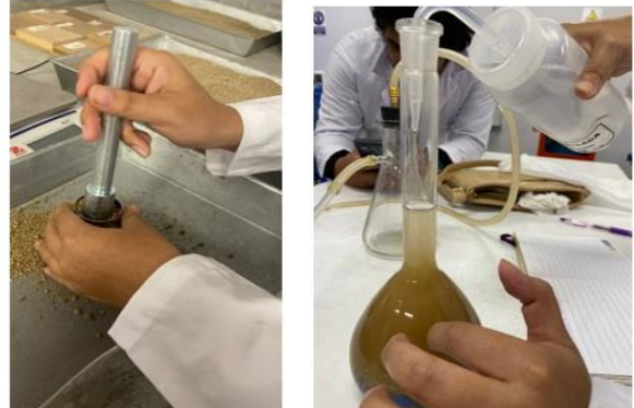
Fig. 9. Peso específico y absorción de agregado fino. (Elaboración propia)
