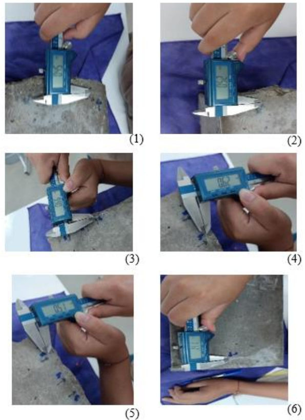
Fig. 14. Fotografías de medición de ancho y largo de grietas en probetas incorporadas con Bacillus subtilis . (Elaboración propia)
