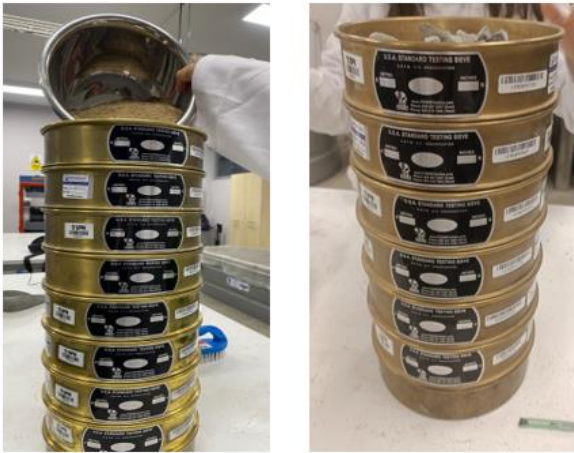
Fig. 4. Tamizado de agregados finos (arena) y gruesos (piedra). (Elaboración propia)
