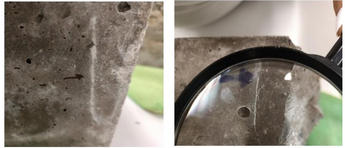
Fig. 13. Fotografías de grietas autorreparadas con Bacillus subtilis mediante la precipitación de calcita. (Elaboración propia)
