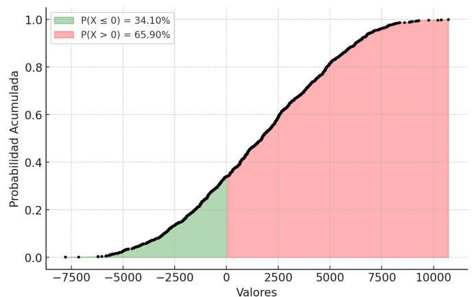
Figura 12 – Función de distribución acumulada (CDF) para los 1000 escenarios simulados
