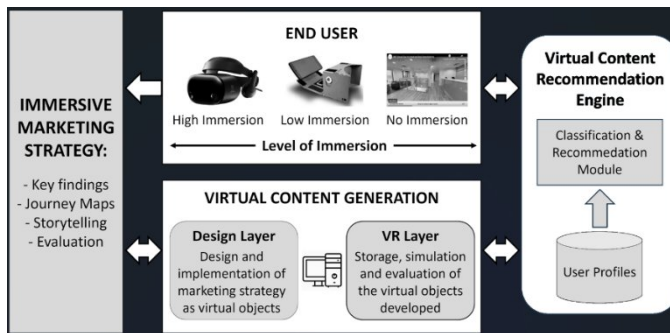
Fig. 4 Arquitectura de software. Fuente: Adaptado de Alfaro, et. al. (2019).
