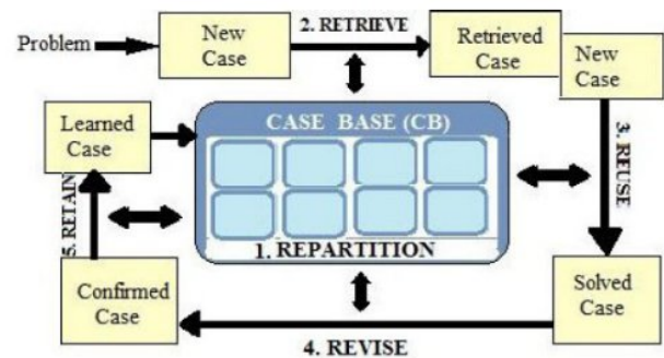
Fig. 2 Ciclo CBR basado
