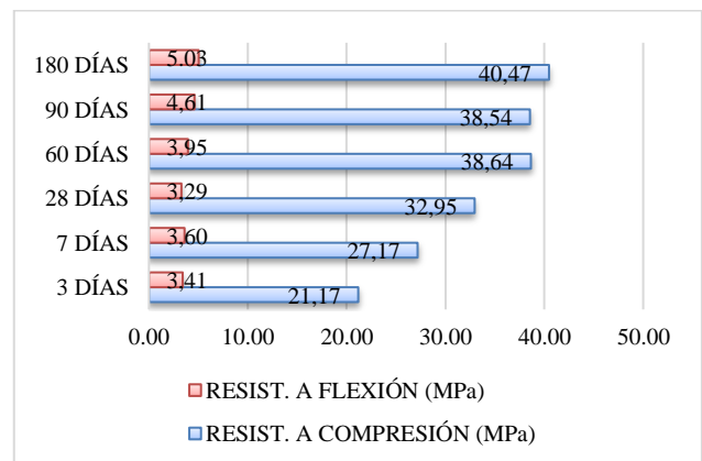
Fig. 2 Gráfica de las resistencias del concreto con 2,50% de aditivo acelerante
