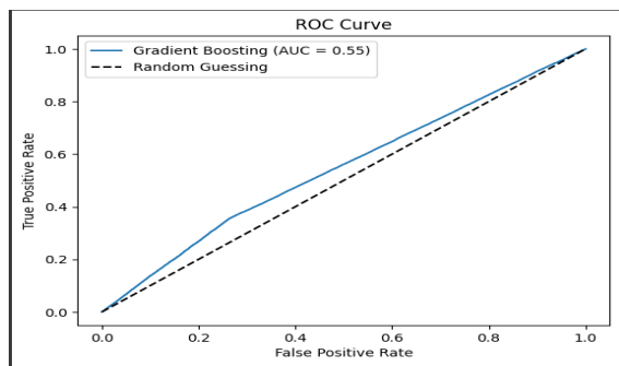
Figura 4: Curva AUC-ROC del Modelo
