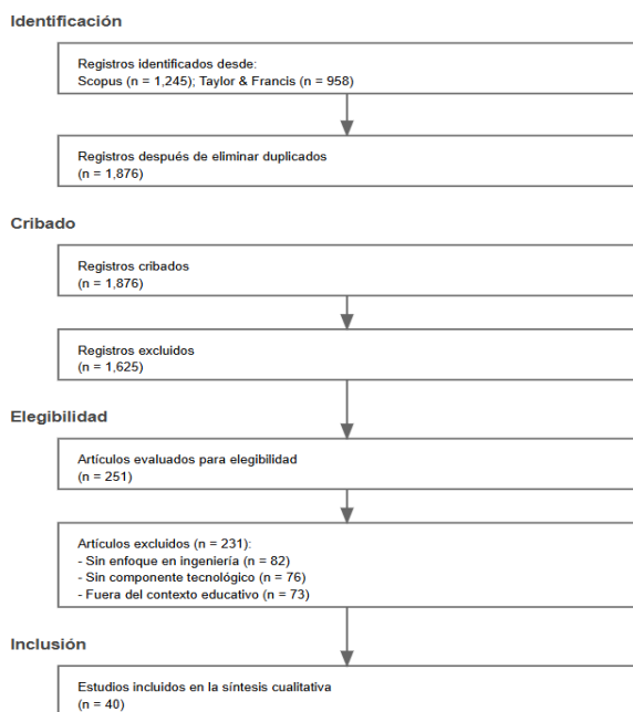
Fig. 1 Análisis PRISMA
