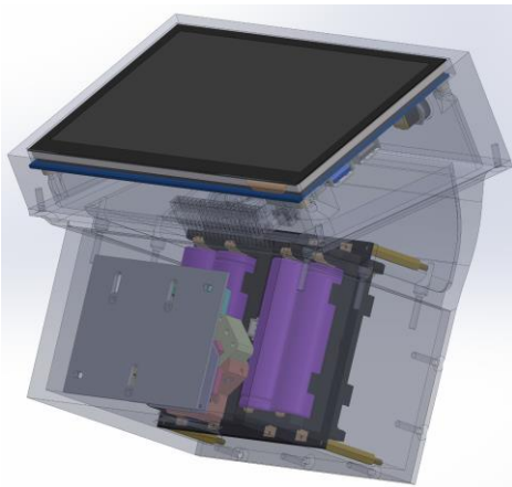
Fig.4 Esquema final del prototipo
