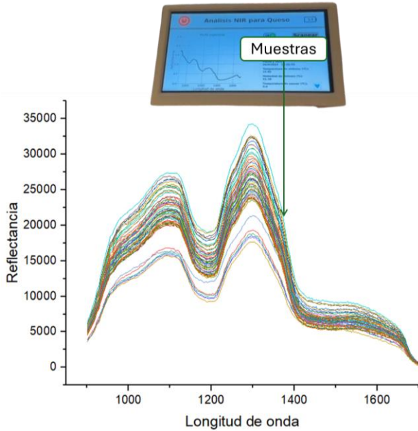
Fig.8 Espectros medidos con equipo prototipo
