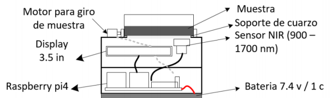
Fig.3 Esquema base del prototipo
