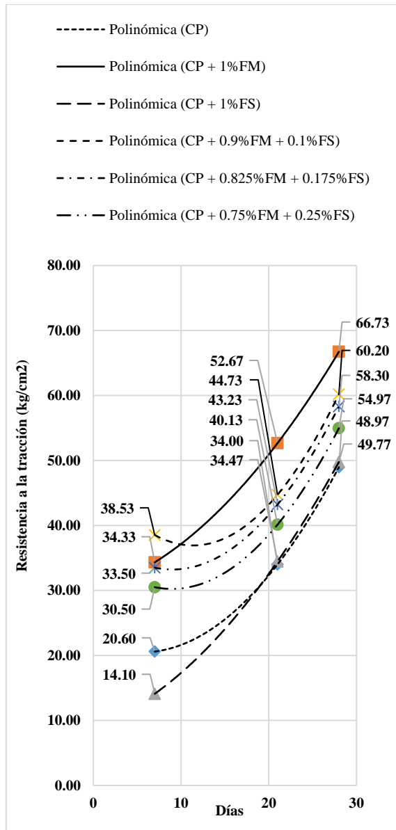
Fig. 3 Resistencia a la tracción del hormigón por tipo de diseños con fibras sintéticas (FS) y fibras metálicas (FM).
