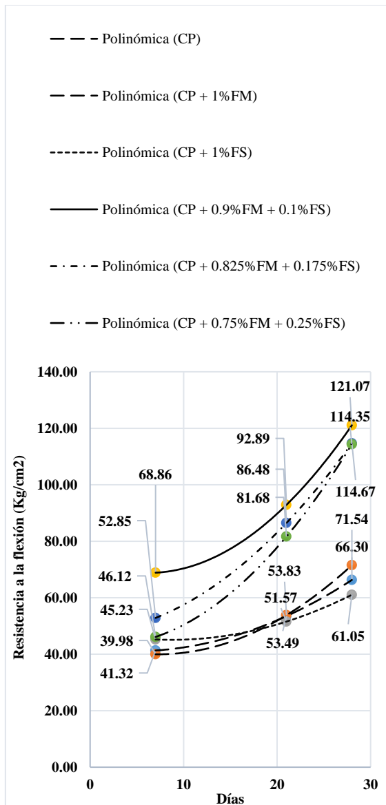
Fig. 2 Resistencia a la flexión del hormigón por tipo de diseños con fibras sintéticas (FS) y fibras metálicas (FM).
