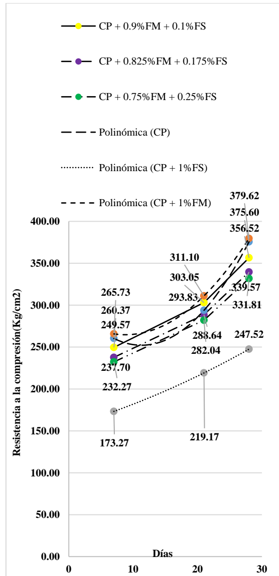
Fig. 1 Resistencia a la compresión del hormigón por tipo de diseños con fibras sintéticas (FS) y fibras metálicas (FM).
