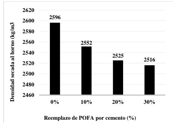
Fig. 4 Resultados de densidad MP, M10%, M20%, M30% a los 28 días.
