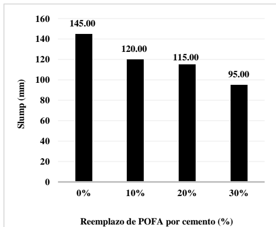
Fig. 1 Resultados del asentamiento para MP, M10%, M20%, M30%.
