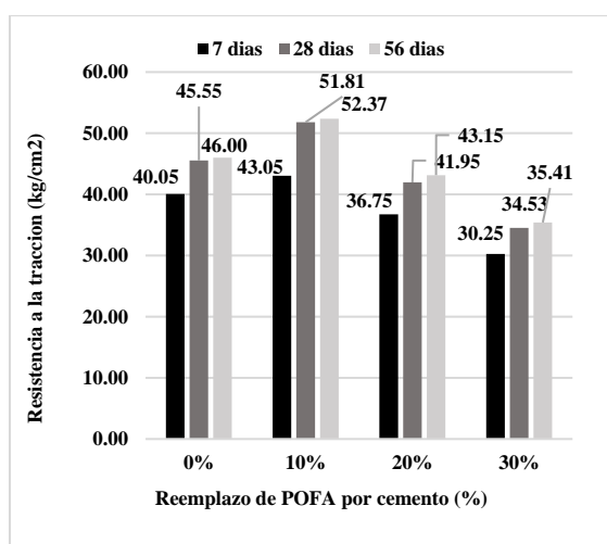
Fig. 3 Resultados de resistencia tracción MP, M10%, M20%, M30% a los 28 días.
