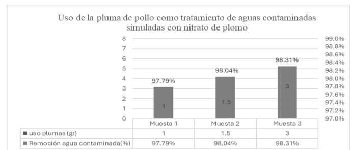
Fig. 5. Uso de la pluma de pollo como tratamiento para la remoción de agua contaminada simulada con nitrato de plomo en la primera repetición.
