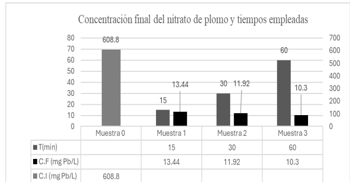
Fig. 3. Concentración final del agua contaminada simulada con nitrato de plomo mediante el uso de la pluma de pollo empleando 15 (min), 30 (min) y 60 (min) de tiempo de contacto para la remoción en la primera repetición.
