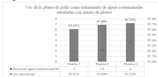
En la Fig. 8 se aprecia que, a más cantidad de pluma usada, el nitrato de plomo en agua disminuye progresivamente, al usar 3 (gr) de plumas de pollo la eficiencia en la remoción del nitrato de plomo alcanzó un máximo del 97.72 (%).
