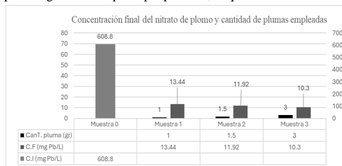
Fig. 1. Concentración final del agua contaminada simulada con nitrato de plomo mediante el uso de la pluma de pollo empleando 1(gr),1.5(gr) y 3 (gr) como tratamiento para la remoción en la primera repetición.
