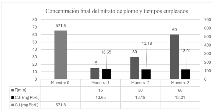
Fig. 4. Concentración final del agua contaminada simulada con nitrato de plomo mediante el uso de la pluma de pollo empleando 15 (min), 30 (min) y 60 (min) de tiempo de contacto para la remoción en la segunda repetición.
