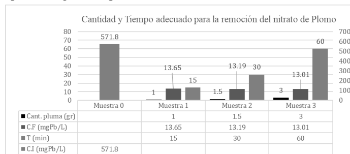
Fig. 2. Cantidad y tiempo adecuado del uso de plumas de pollo empleando 1(gr),1.5(gr) y 3(gr) como tratamiento para la segunda repetición.
