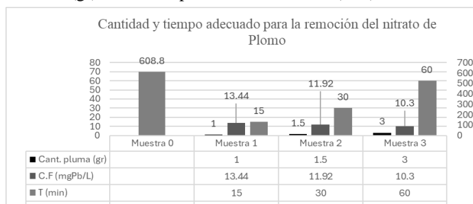
Fig. 1. Cantidad y tiempo adecuado del uso de plumas de pollo empleando 1(gr),1.5(gr) y 3 (gr) como tratamiento para la remoción en la primera repetición
