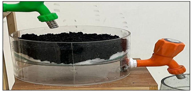
Fig. 8 Prototipo de la última fase con rejilla divisora, malla de micrón, algodón y carbón activado.
