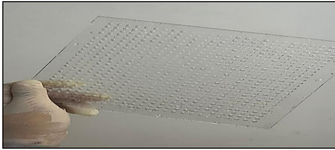
Fig. 6 Rejilla de divisora de cada filtro. Nota. Divisor de acrílico con agujeros de 0.5 mm.
