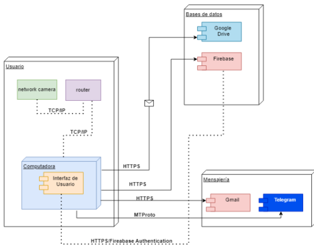
Fig. 6 Diagrama de Despliegue
