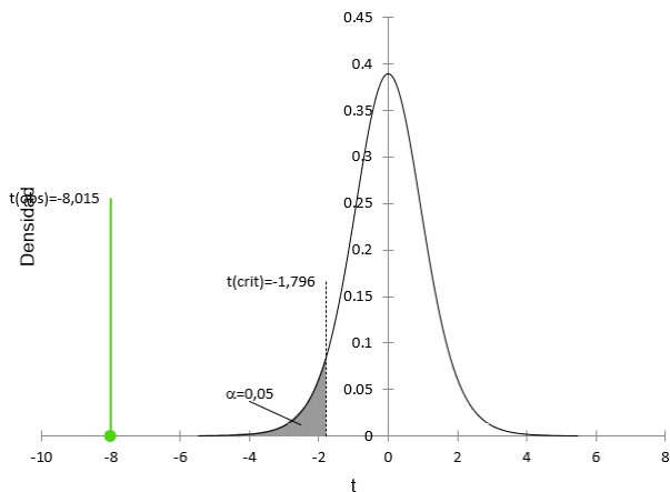
Fig. 15 Evaluación del área de aceptación o rechazo del porcentaje de Precisión
