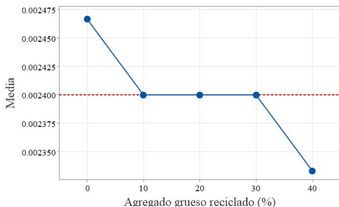
Fig. 3 Efectos principales para densidad (kg/cm 3 )
