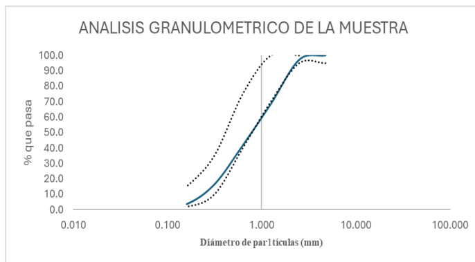
Fig. 1 Curva granulométrica del agregado [1].
