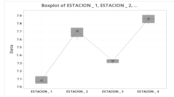
Figura 3 Gráfica de caja de pH entre Estaciones
