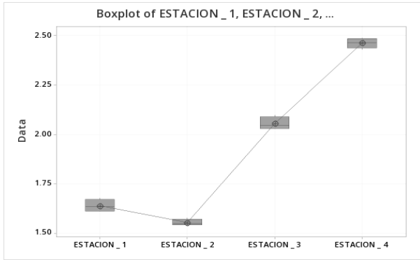
Figura 5 Gráfica de caja de Oxígeno Disuelto entre Estaciones
