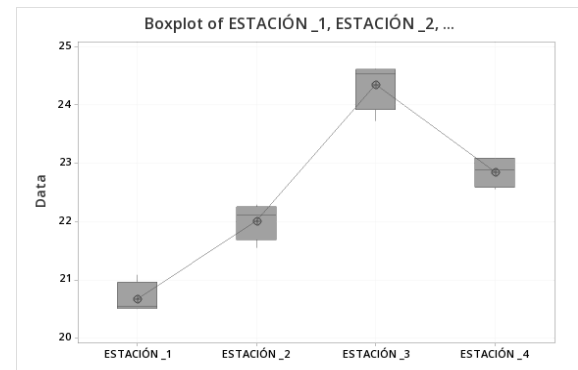
Figura 4 Gráfica de caja de Temperatura entre Estaciones
