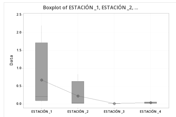
Figura 8 Gráfica de Fósforo Total entre Estaciones
