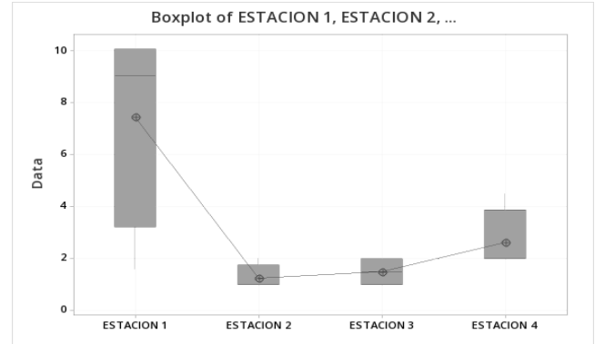
Figura 7 Gráfica de caja de DBO5 entre Estaciones
