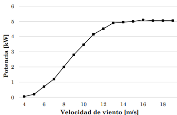
Fig. 2 Curva de potencia versus la velocidad del viento para la turbina Eevance-5000 [17].
