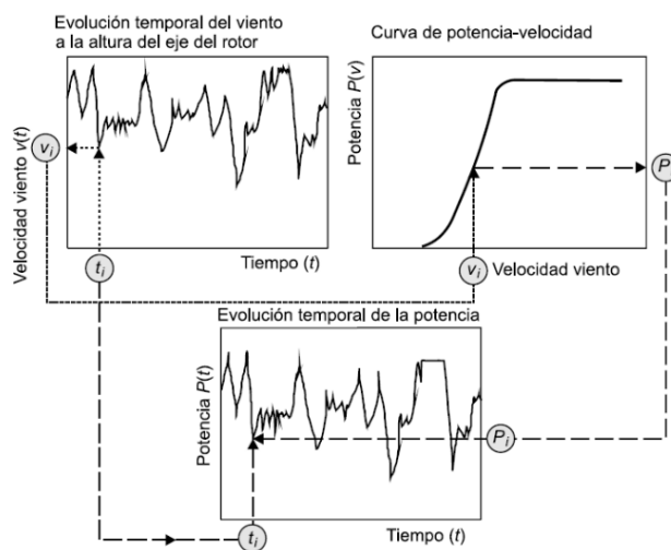
Fig. 3 Proceso de cálculo de la potencia total generada [19].
