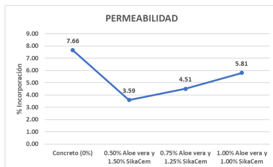
Figura 6. Permeabilidad del concreto
