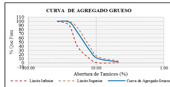
Figura 1. Curva granulométrica de agregado grueso
