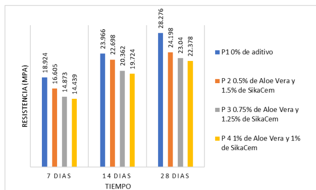
Figura 2. Resultados de ensayos de compresión
