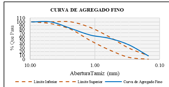
Figura 3. Curva granulométrica de agregado fino
