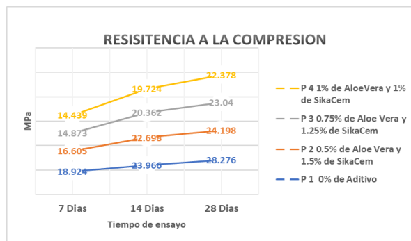
Figura 4. Representación de resistencia a la compresión
