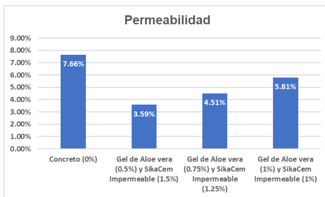
Figura 3. De permeabilidad de los diferentes diseños de concreto.
