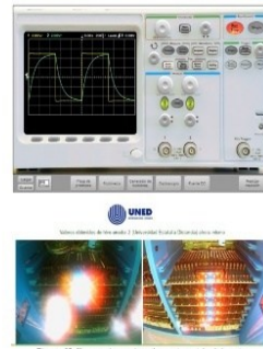
Figura 10. Respuesta en el osciloscopio y vista del equipo
