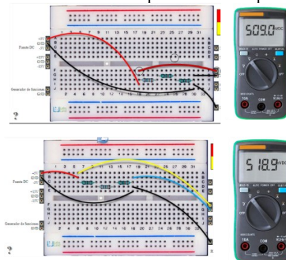
Fig. 9. Resultados de mediciones al circuito divisor de voltaje
