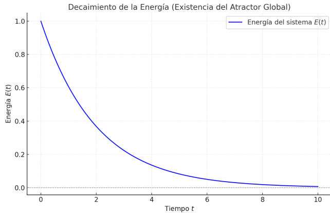
Figura 4: Decaimiento exponencial de la energía E(t) con respecto al tiempo t .
