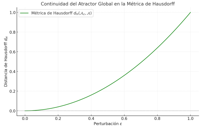
Figura 5: Convergencia de la distancia de Hausdorff d_H(\mathcal{A}_\varepsilon, \mathcal{A}) .
