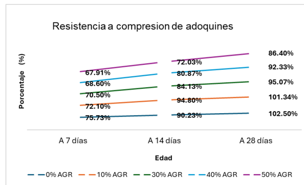
Fig. 5. Grafica resistencia a compresión de diseño 28MPa en adocuin con sustitución parcial de 10%, 30%, 40% y 50% de ARG.
