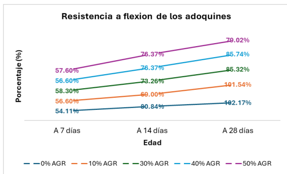
Figura 7. Resultado resistencia a flexión de diseño 28MPa en adoquín con sustituciones parciales del agregado grueso natura por ARG
