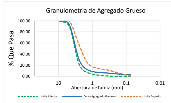
Figura 3. Granulometría de A. F
