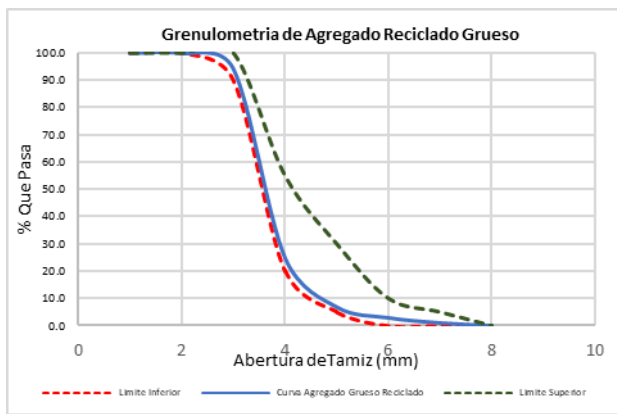
Fig. 4. Granulometría de ARG.
