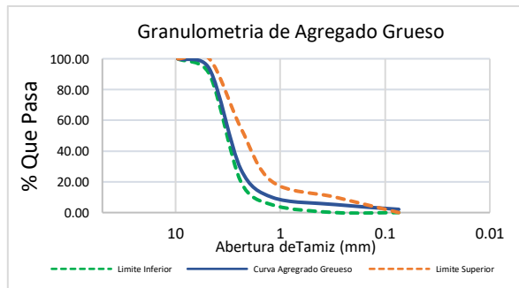
Fig. 2. Granulometría de A. G
