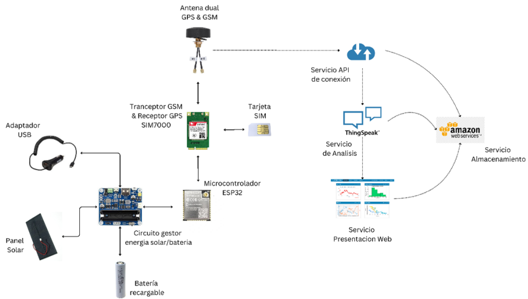
Fig. 2: Componentes del sistema propuesto.
