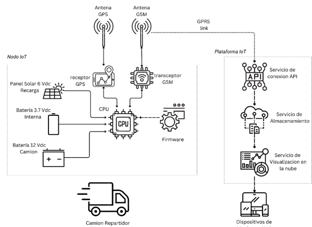
Fig. 1: Arquitectura del sistema propuesto.
