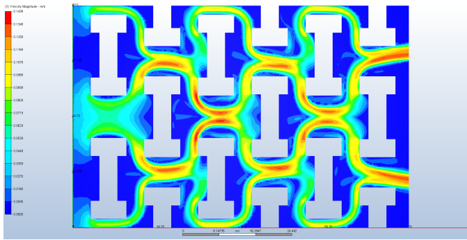
Fig. 6 Simulación de velocidad a 0.0101 m/s
