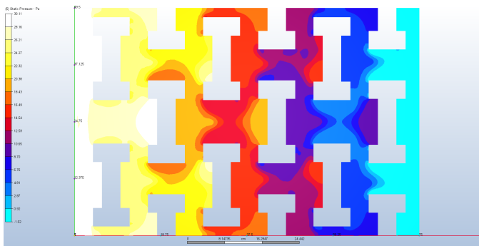
Fig. 7 Simulación de presión a 0.0101 m/s
