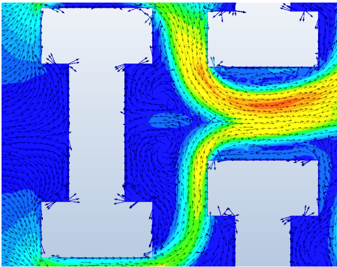
Fig.13 Velocidad vector para caso turbulento
