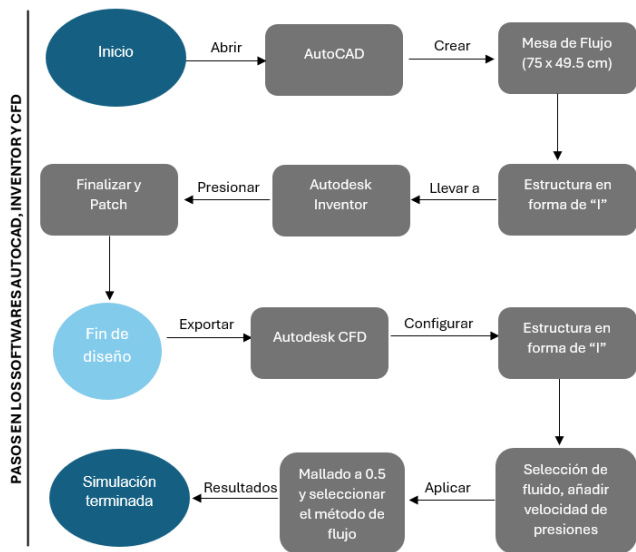
Fig.4 Flujograma de pasos en el software AutoCAD, Autodesk Inventor y CFD.
