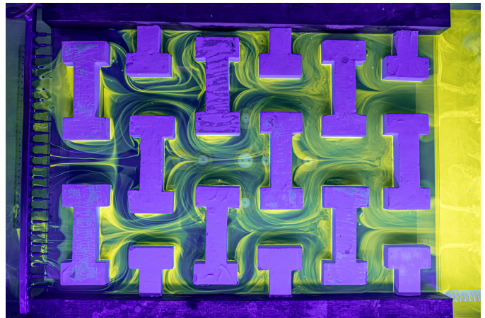
Fig.9 Simulación en la mesa de flujo para el caso laminar
