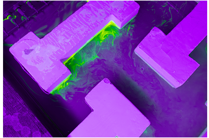
Fig.15 Formación de remolinos
