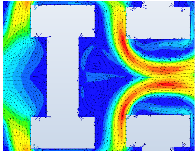
Fig.8 Velocidad vector para caso laminar
