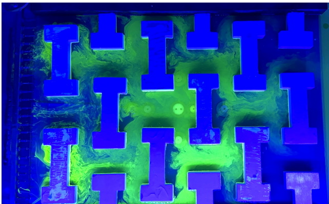
Fig. 14 Movimiento del flujo turbulento
