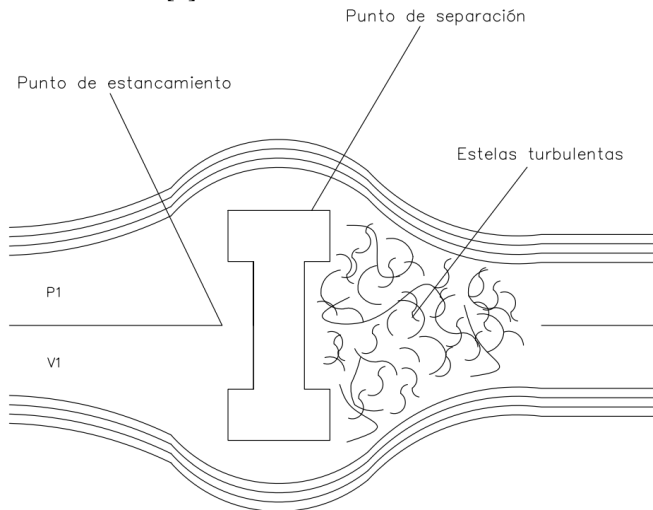
Fig. 1 Punto de estancamiento
