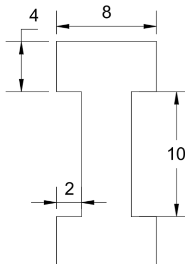
Fig.2 Medidas de la estructura en forma de “I”.
