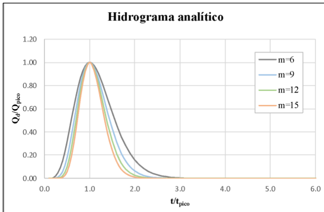
Fig. 1 Hidrograma analítico a través de ecuación matemática
