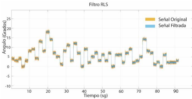
Figura 12: Señal filtrada
