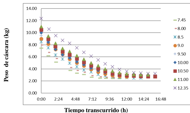
Fig. 3- Curvas de secado al ambiente de las cáscaras de uva Quebranta obtenidas luego de la etapa de pre-fermentación
