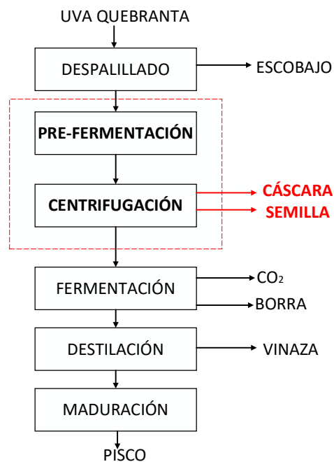
Fig. 1- Diagrama de Bloques de Proceso de la elaboración de Pisco de Uva Quebranta mediante la etapa de pre-fermentación.
