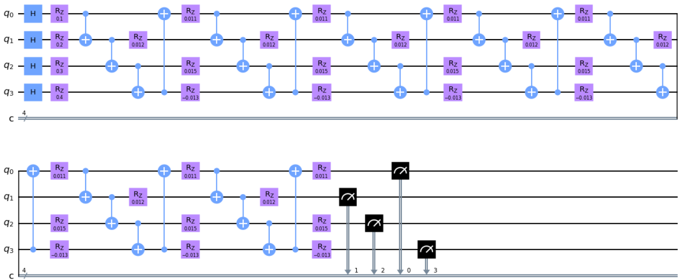
Fig. 6 Capas Variacionales con Capas Entangler Básicas para cuatro Qubits y una Profundidad de 7 Capas, con Puertas CNOT y Rotaciones de Qubit Simple Puertas R_z .
