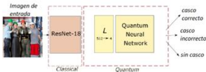
Fig. 8 El modelo de aprendizaje de transferencia cuántica con la Computación Clásica de ResNet-18 y la Computación Cuántica de la Red Neuronal Cuántica.
