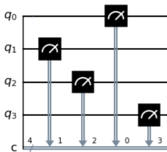
Fig. 7 Capa de Medida con 4 Operadores Pauli Z .
