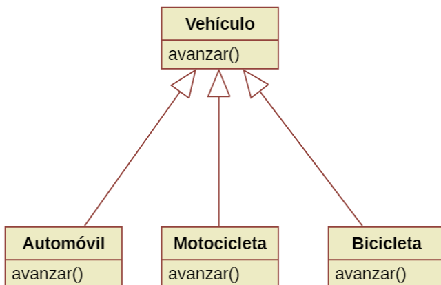
Fig. 21 Diagrama de clases considerando Herencia y Polimorfismo. Método polimórfico “avanzar”
