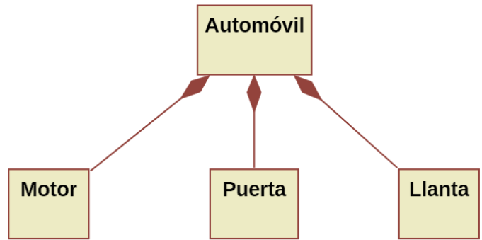
Fig. 18 Diagrama de clases considerando el Automóvil (clase todo) y sus partes (clases parte)
